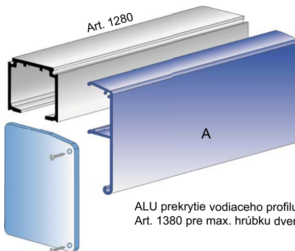
Bočná krytka Art. 89
