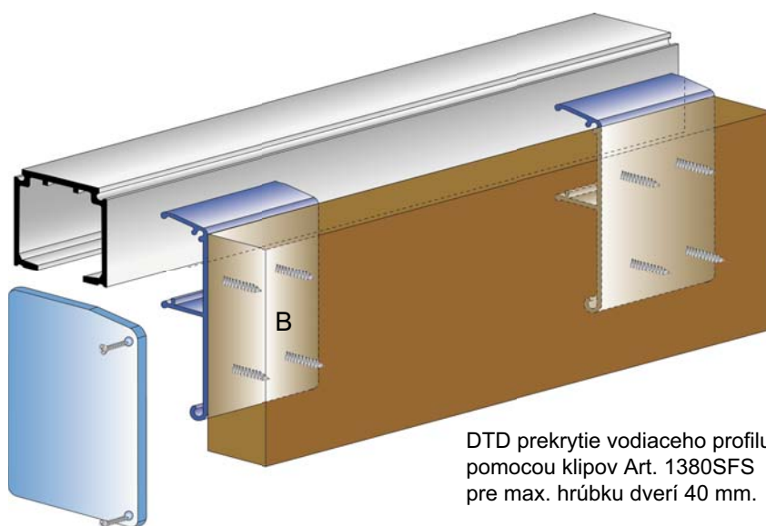
Bočná krytka Art. 89
