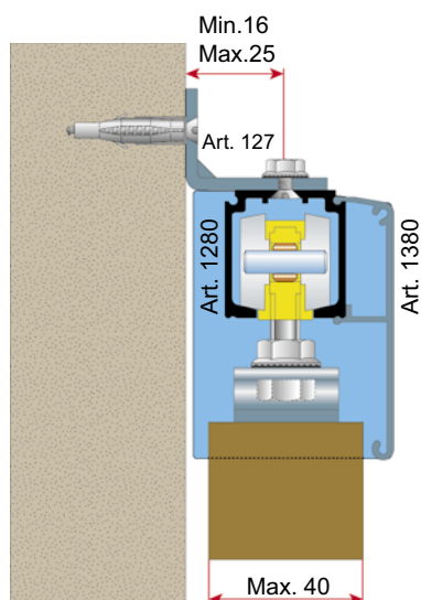
Montáž na stenu ALU prekrytie vodiaceho profilu
