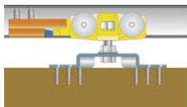
Štandardná montáž vozíka NR
