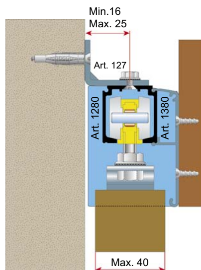
Montáž na stenu DTD prekrytie vodiaceho profilu
