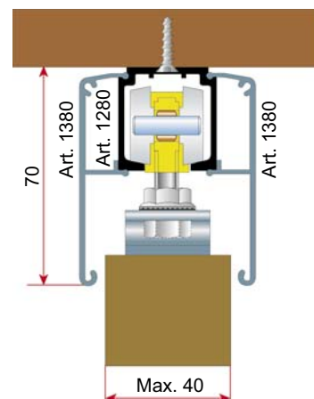
Montáž do stropu ALU prekrytie vodiaceho profilu
